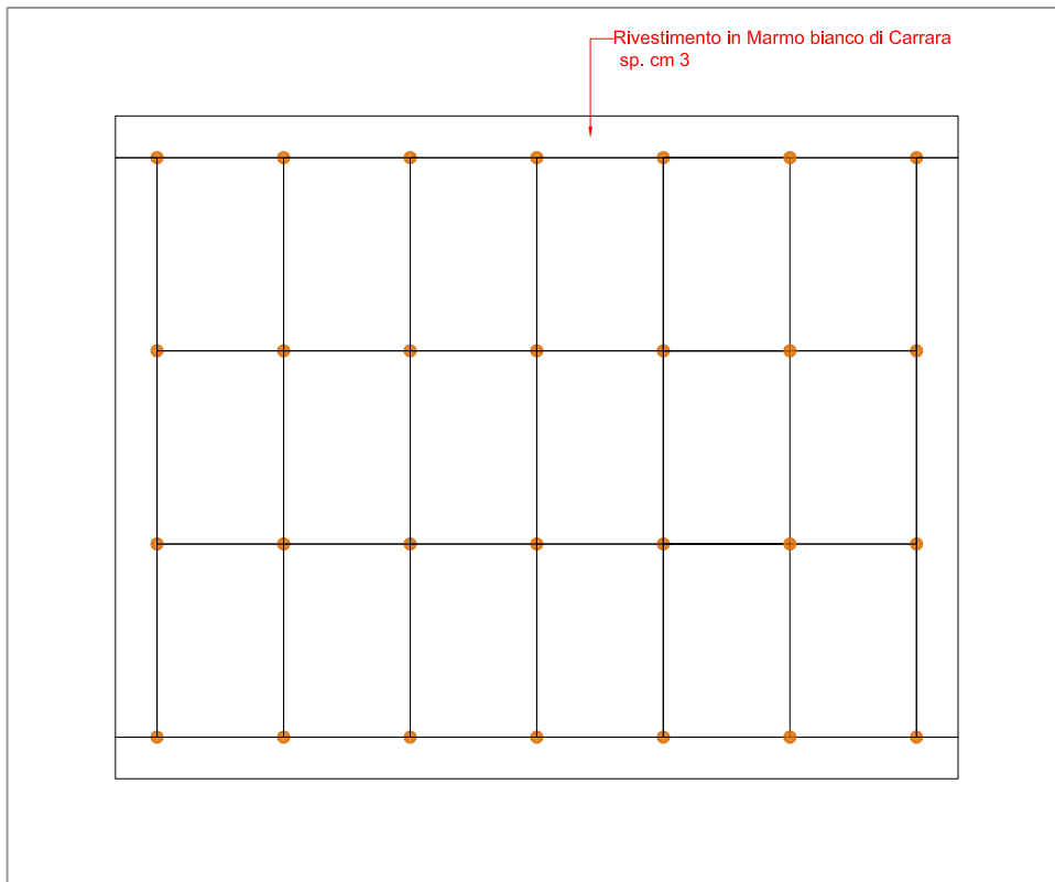
Prospetto laterale
