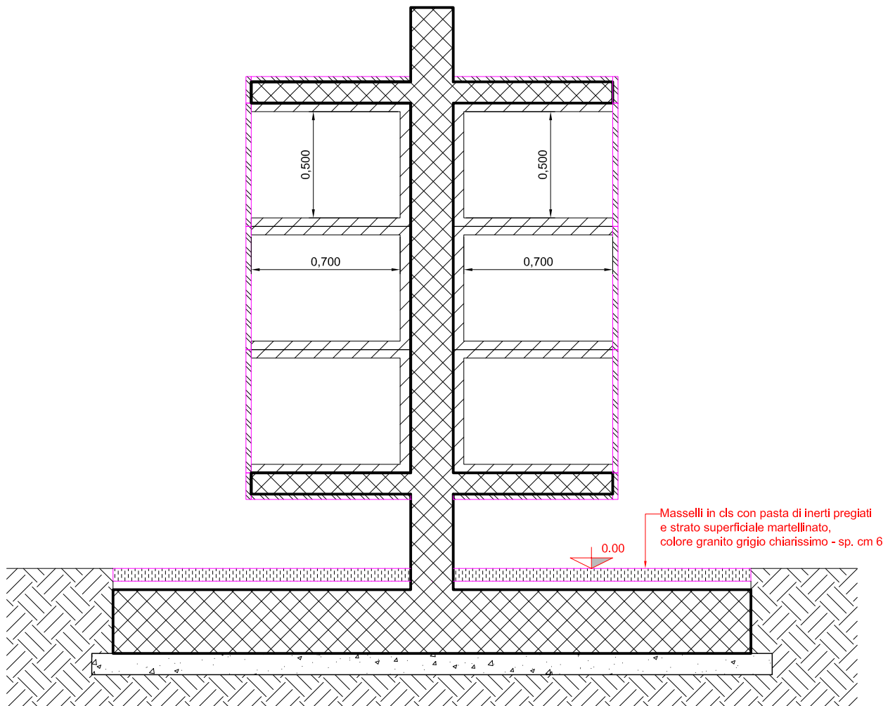
Sezione trasversale
